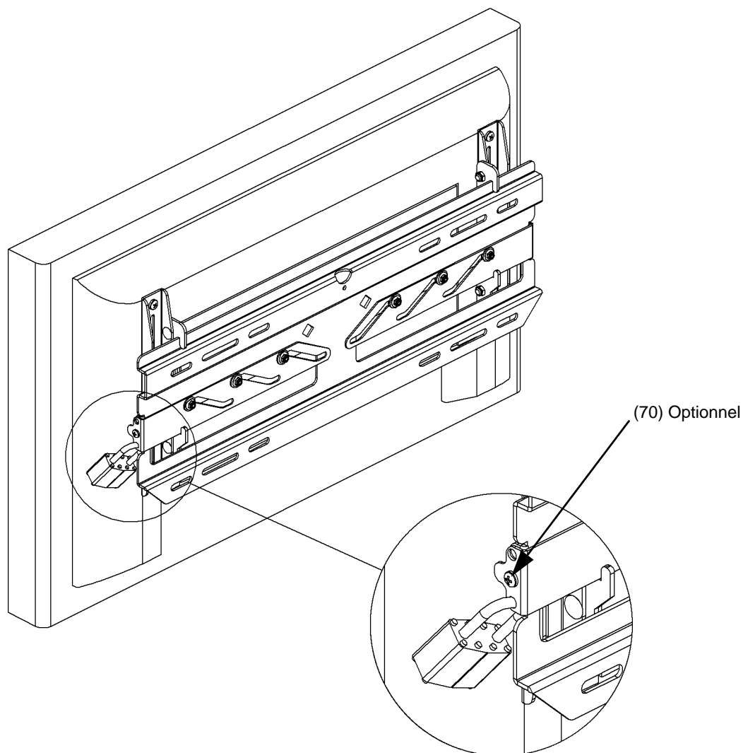
Figure 9. Sécuriser l'écran
